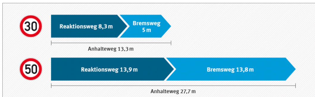
Abb. 3: Anhalteweg bei Tempo 30 und bei Tempo 50 (Quelle: UBA)
